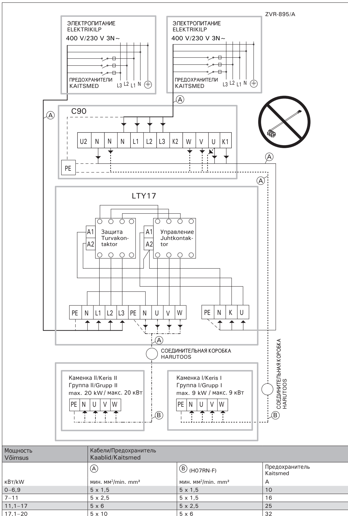
Рисунок 8. Подключение дополнительного блока питания LTY17 с пультом управления C90 Joonis 8. Lisakontaktori LTY17 ühendamine juhtimiskeskuse C90-ga
