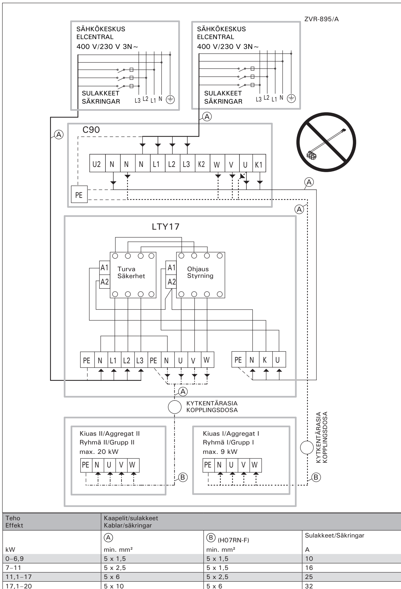
Kuva 8. LTY17 lisätehoyksikön kytkentä C90 ohjauskeskuksen kanssa Bild 8. Koppling av extra effektenheten LTY17 till styrenheten C90
