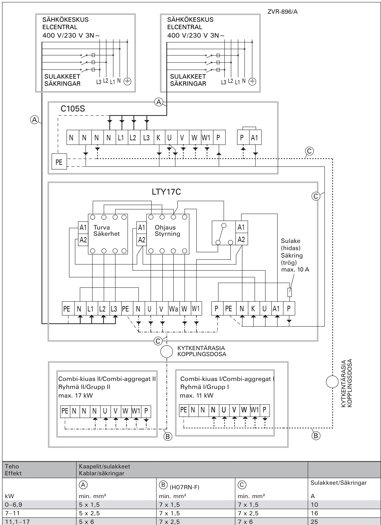
Kuva 14. LTY17C lisätehoyksikön kytkentä C105S ohjauskeskuksen kanssa
