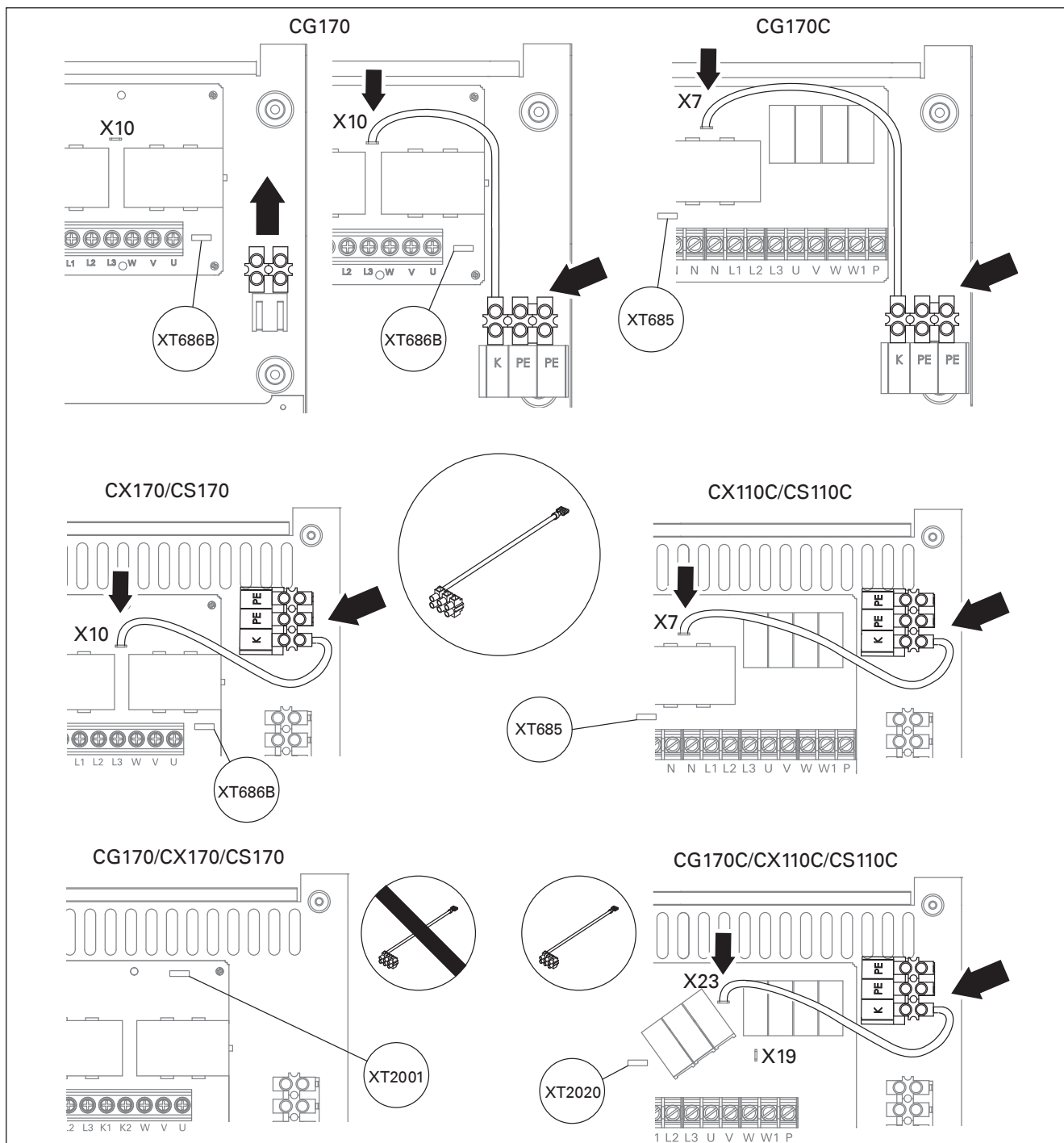
Рисунок 4. Подключение дополнительной клеммной колодки внутри блока питания пульты управления CG170/CG170C/CX170/CX110C/CS170/CS110C
