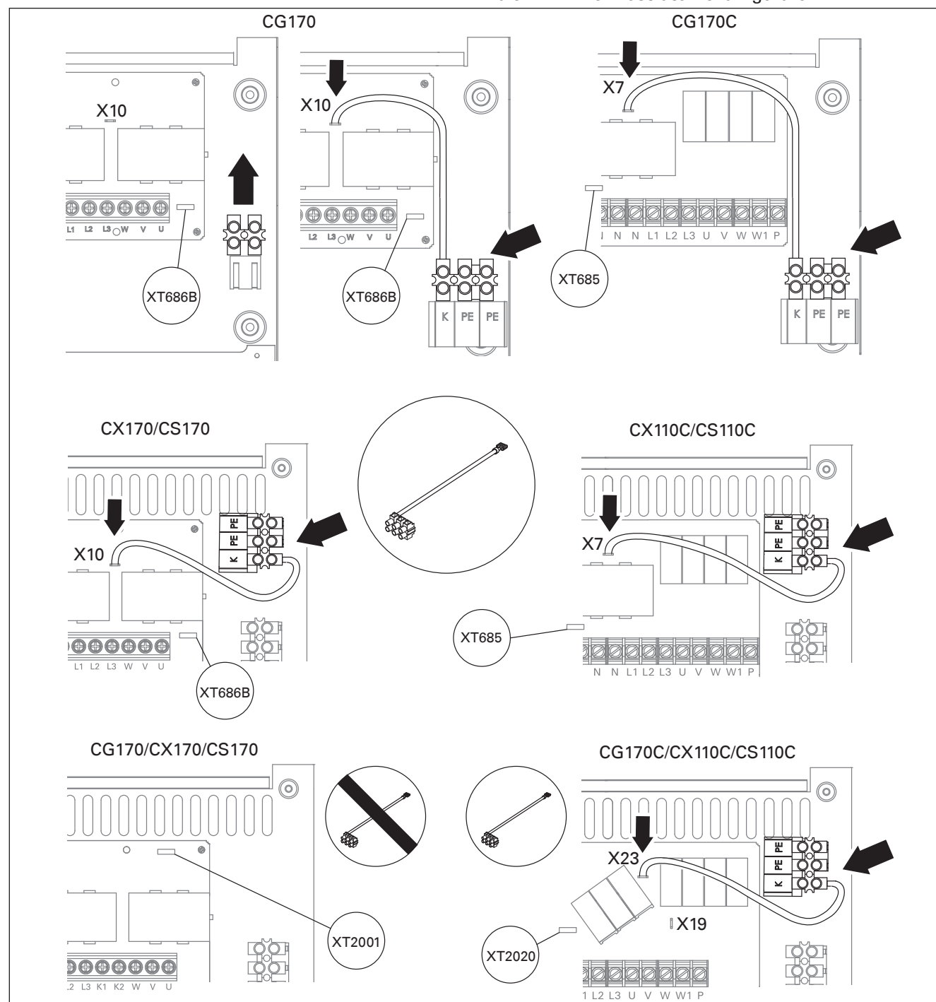
Figura 4. Collegamento della morsettiere supplementare nella centralina CG170/CG170C
