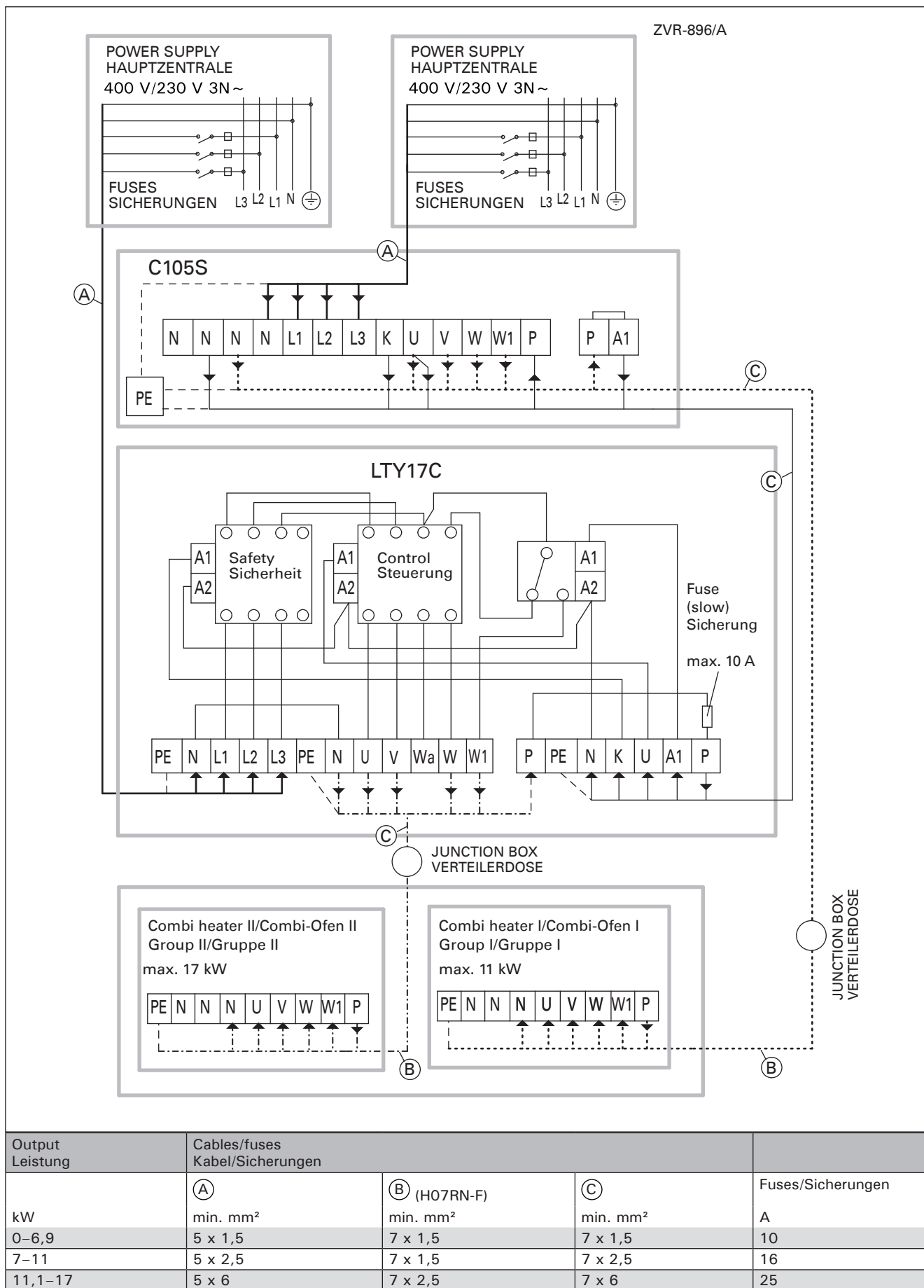
Figure 14. Connection of power extension unit LTY17C with control unit C105S Abbildung 14. Anschluss der optionalen Leistungseinheit LTY17C mit Steuergerät C105S
