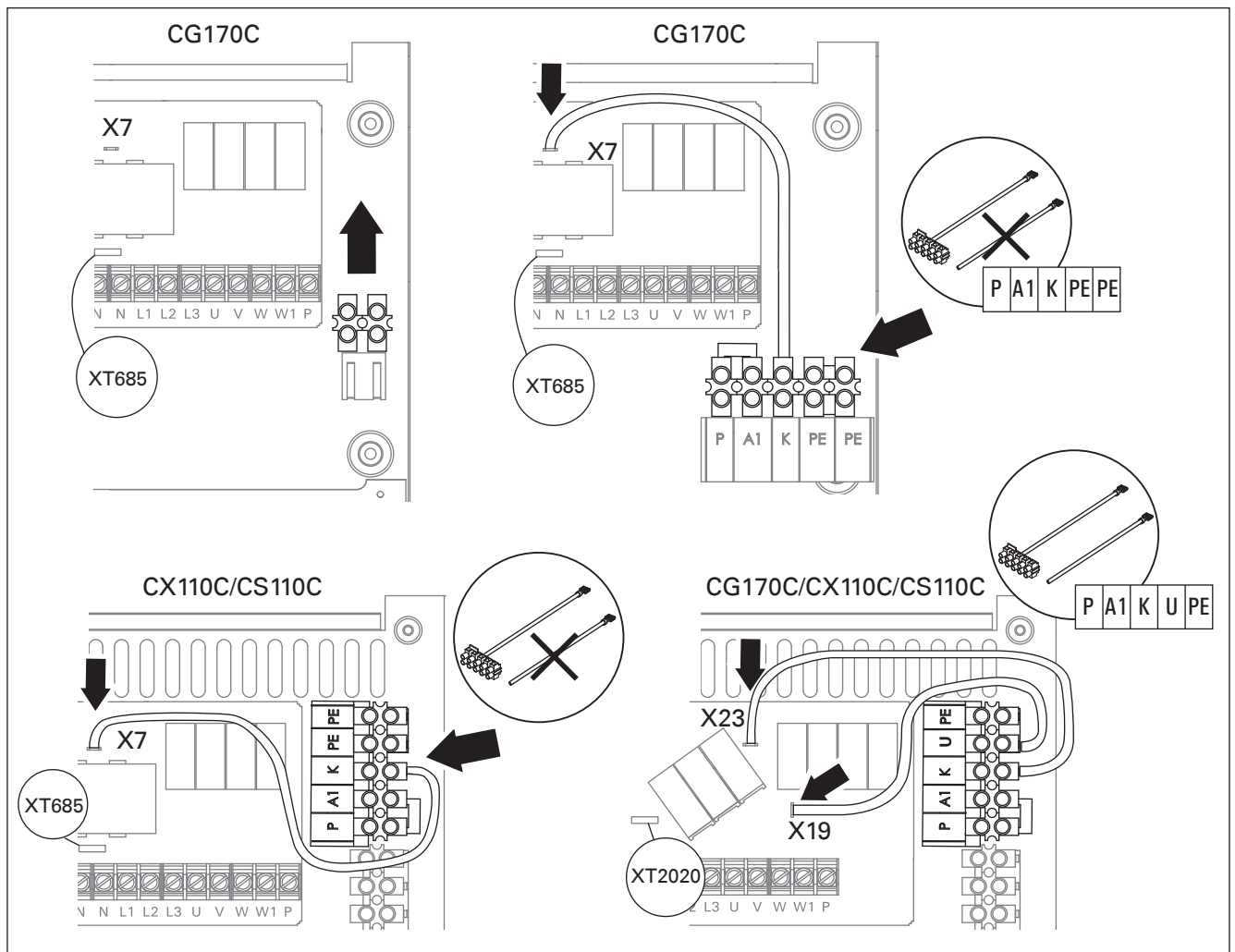
Figura 11. Collegamento della morsettiera supplementare nella centralina CG170C/CX110C/CS110C
