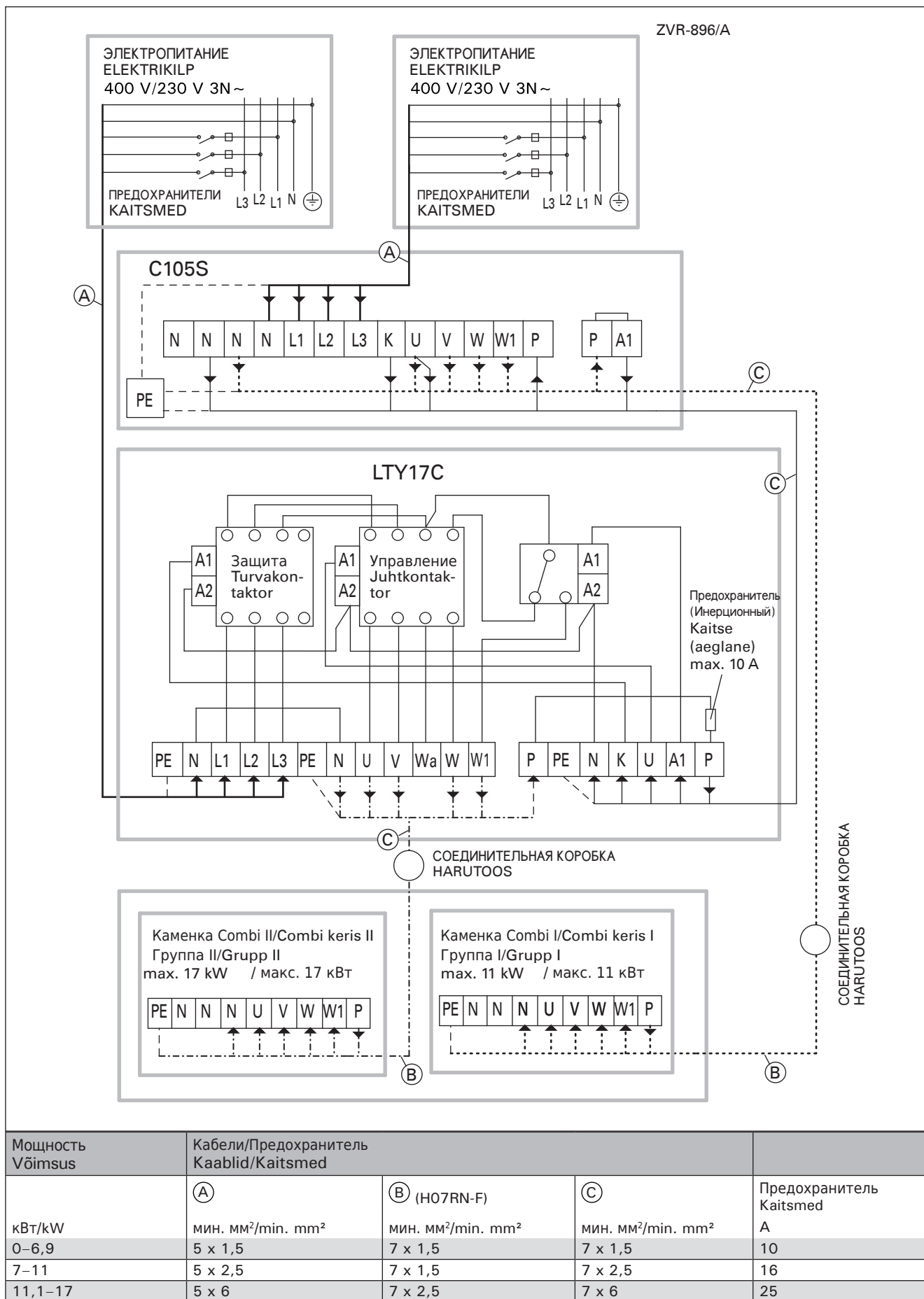
Рисунок 14. Подключение дополнительного блока питания LTY17C с пультом управления C105S Joonis 14. Lisakontaktori LTY17C ühendamise juhtimiskeskuse C105S-ga
