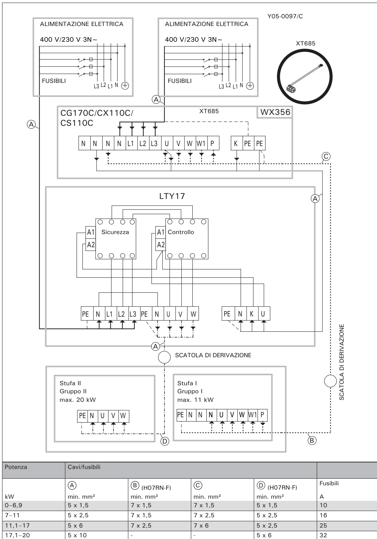
Figura 9. Collegamento dell'unità di alimentazione supplementare LTY17 con la centralina CG170C, CX110C o CS110C (XT685)
