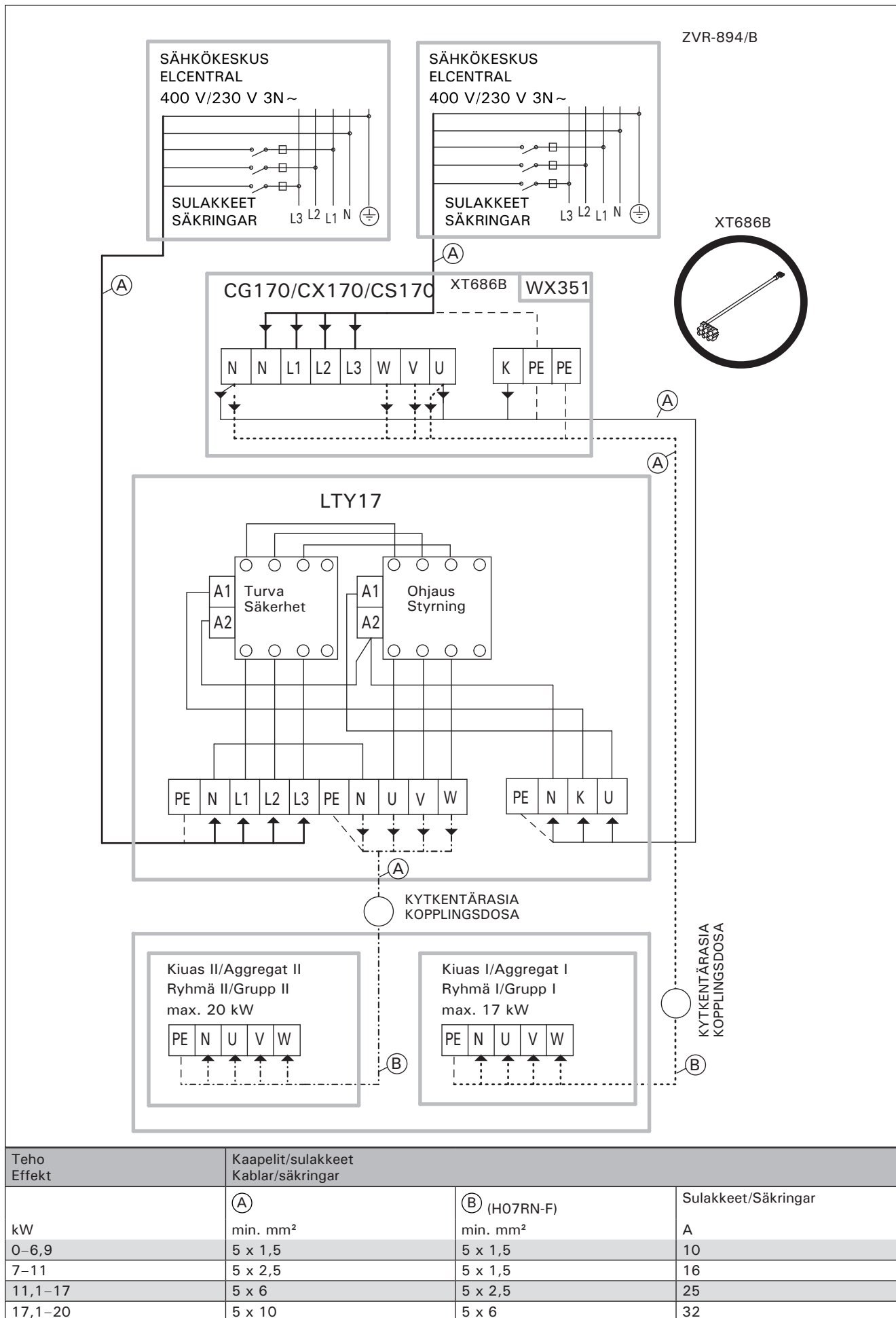
Kuva 6. LTY17 lisätehoyksikön kytkentä CG170, CX170 tai CS170 ohjauskeskuksen kanssa (XT686B). Bild 6. Koppling av extra effektenheten LTY17 till styrenheten CG170, CX170 eller CS170 (XT686B).
