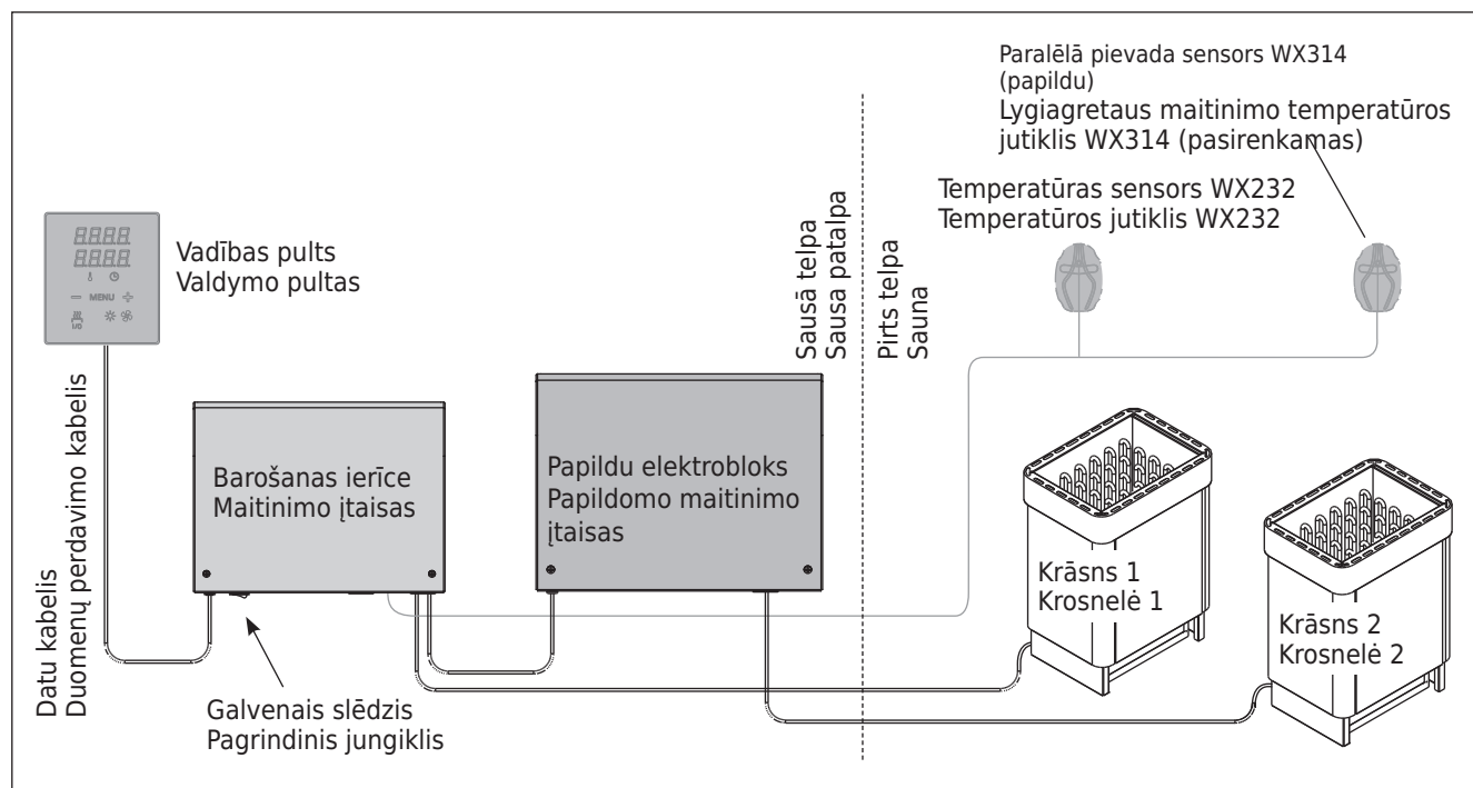
3. zīm. 3 pav. Divu krāšņu paralēlais pievads Dviejų krosnelių lygiagretus maitinimas
