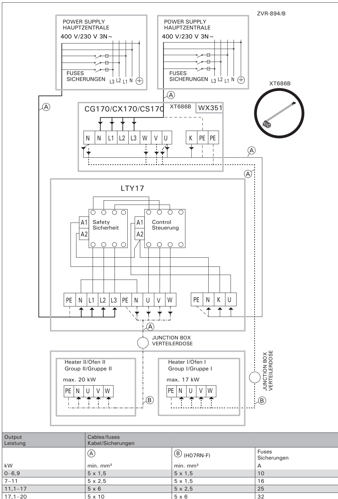
Figure 6. Connection of power extension unit LTY17 with control unit CG170, CX170 or CS170 (XT686B) Abbildung 6. Anschluss der optionalen Leistungseinheit LTY17 mit Steuergerät CG170, CX170 oder CS170 (XT686B)
