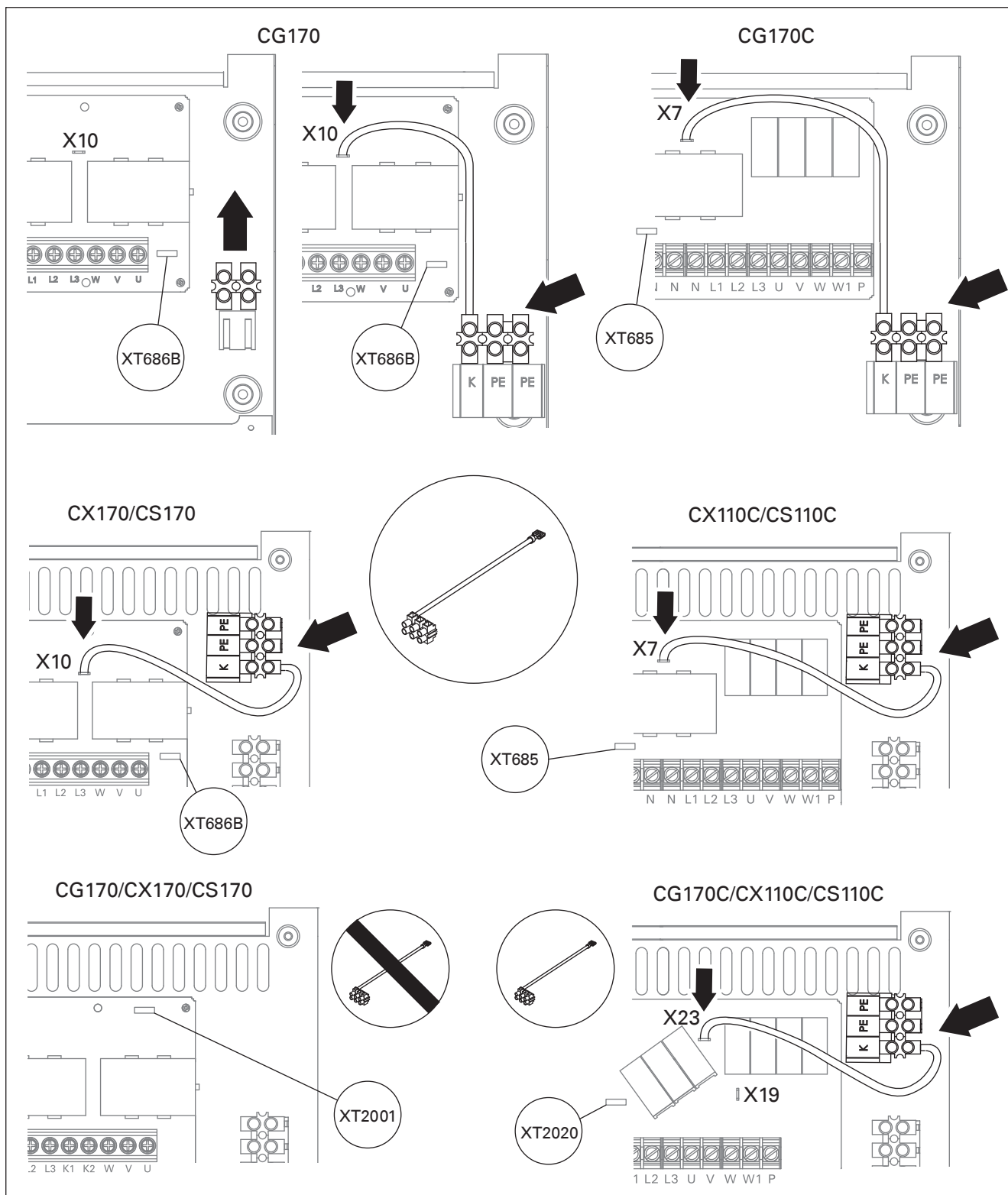
4. zīm. Papildu spaiļu bloka pievienošana barošanas ierīces CG170/CG170C/CX170/CX110C/CS170/CS110C iekšpusē 4 pav. Papildomas gnybtu rīklēs prijungimas valdymo pults CG170/CG170C/CX170/CX110C/CS170/CS110C viduje
