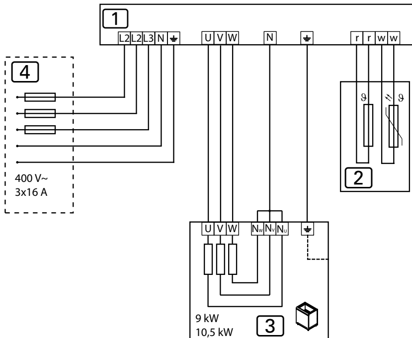
Bild 3 Kopplingsschema för Qube 9 kW och 10,5 kW (QUBE-090/QUBE-105)
