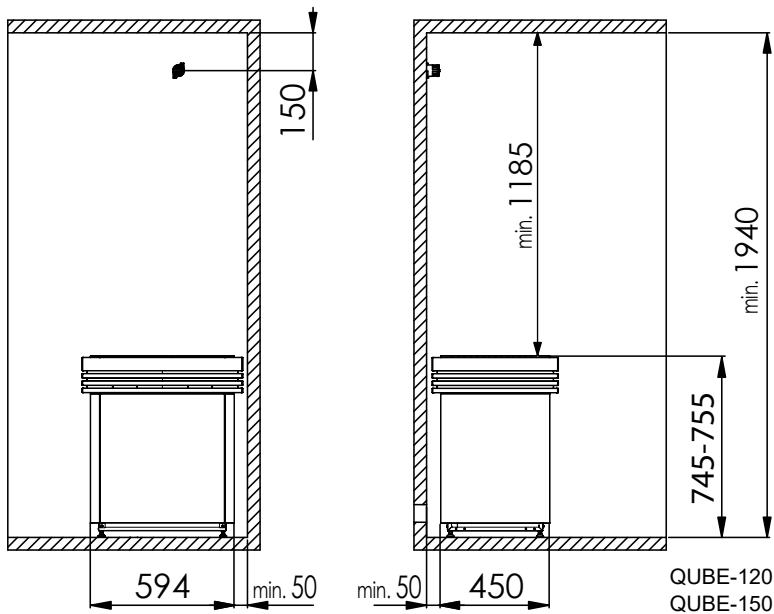
afb. 2 Veiligheidsafstanden Qube 12 kW en 15 kW (QUBE-120 / QUBE-150) Afmetingen in mm
